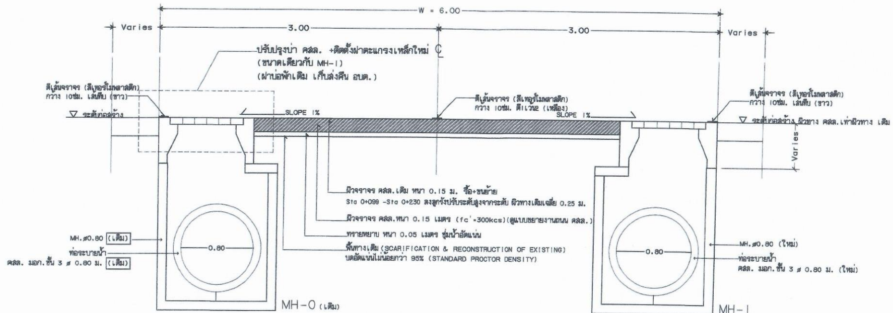
รูปตัดโครงสร้างทาง 1-1 มาตราส่วน 1:30
