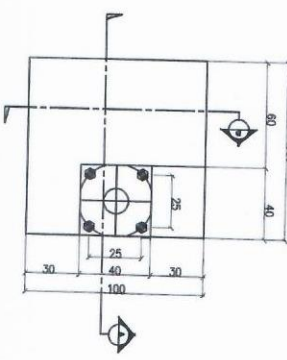
ฐานเสาไฟฟ้าแบบที่ 2
