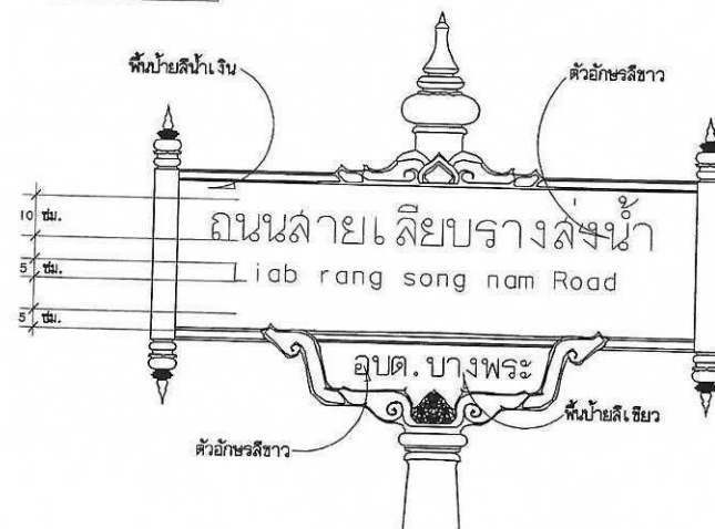
รูปแสดงป้ายชื่อถนน ป้ายแบบที่ ②
