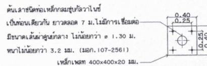
รายละเอียด STEEL BASE PLATE
