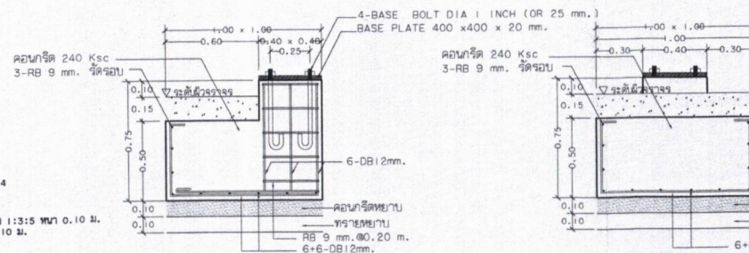
รูปตัด B-B
