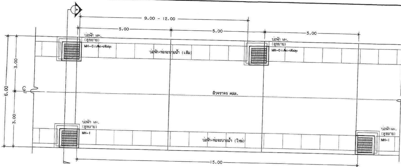
แปลนถนน คลส. + ท่อระบายน้ำ มาตราส่วน 1:75
