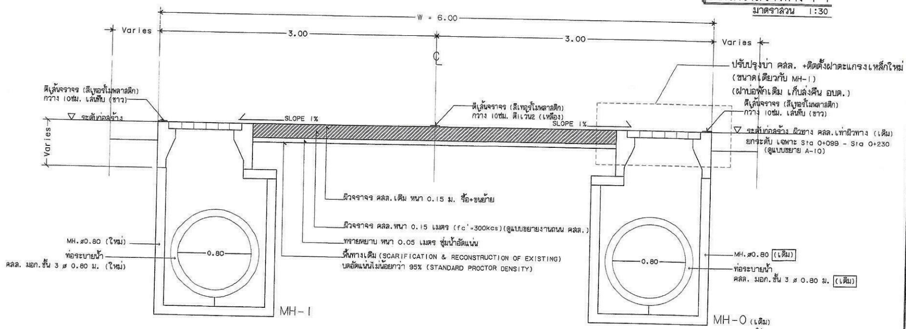
รูปตัดโครงสร้างทาง 2-2 มาตราส่วน 1:30
