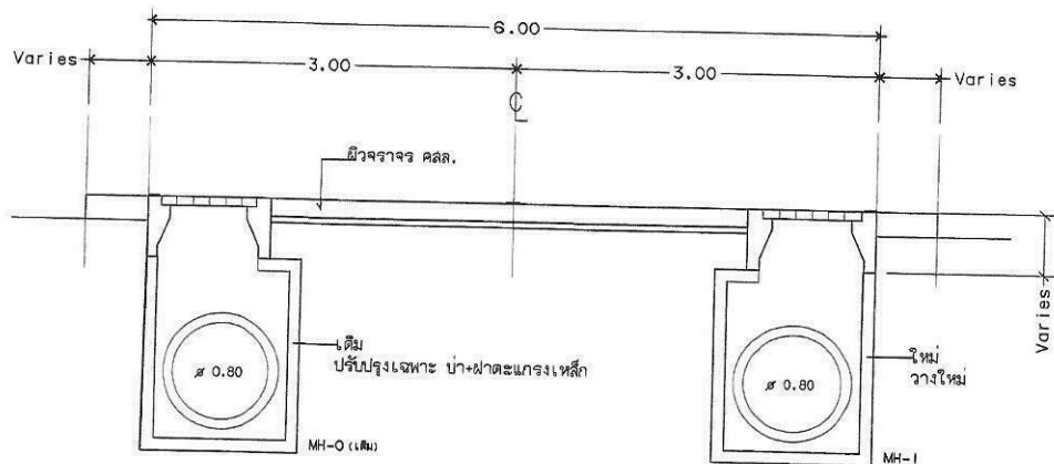
รูปตัด A-A มาตราส่วน NTS
