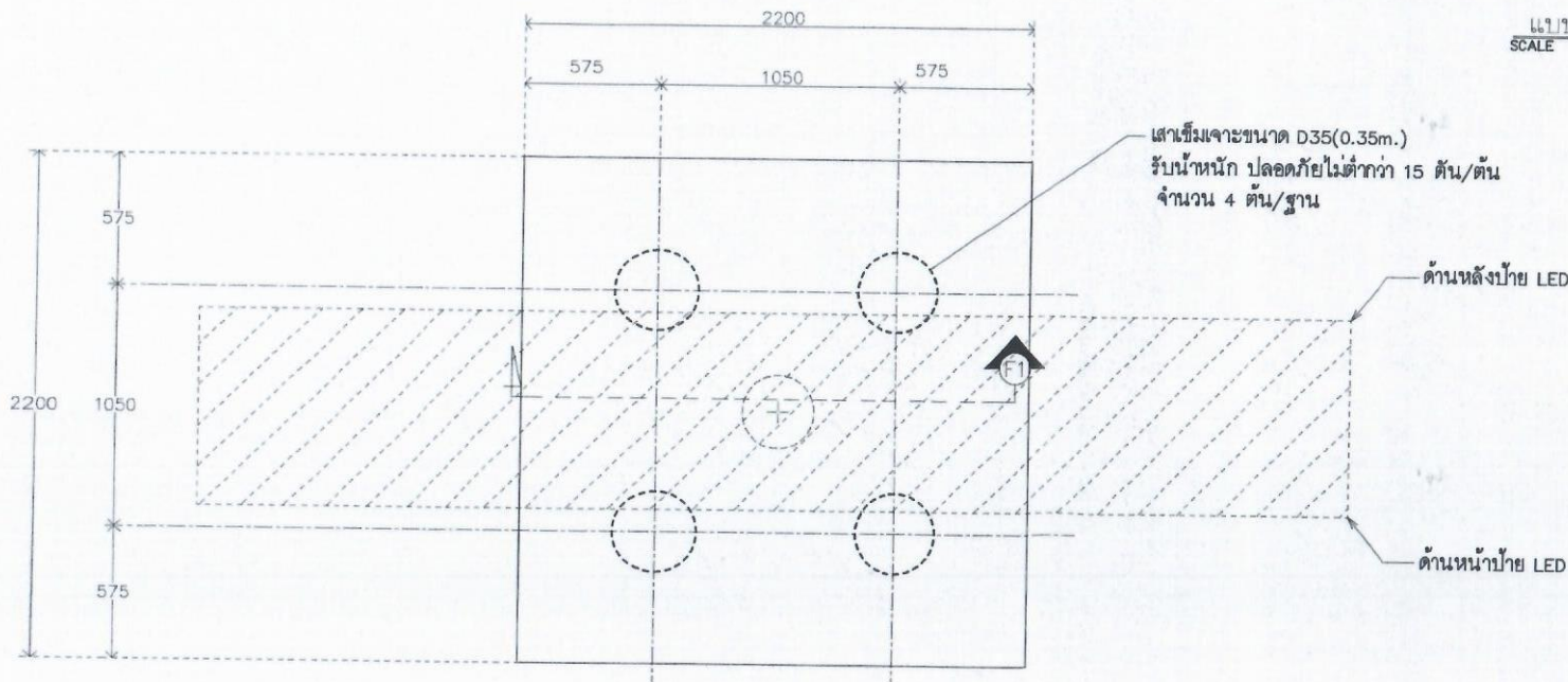
FOOTING F1 SCALE 1:25
