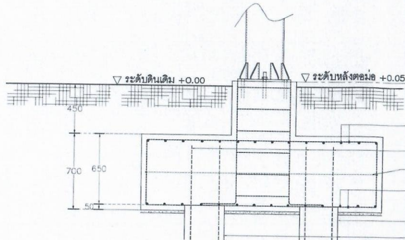
SECTION F1 SCALE 1:25
