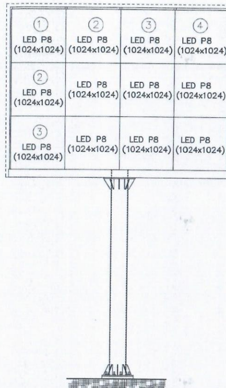
รูปด้านหน้า SCALE 1 : 50
