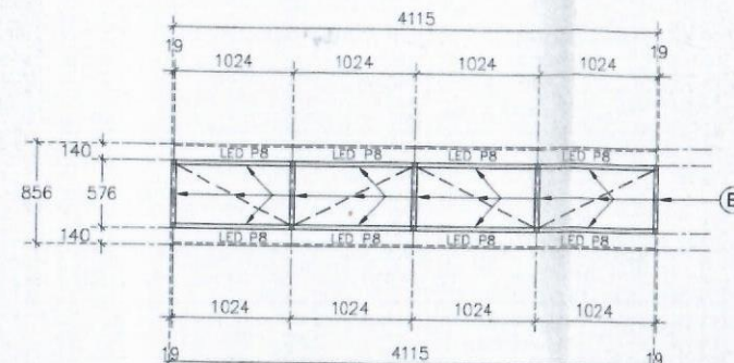
SECTION E SCALE 1 : 50
