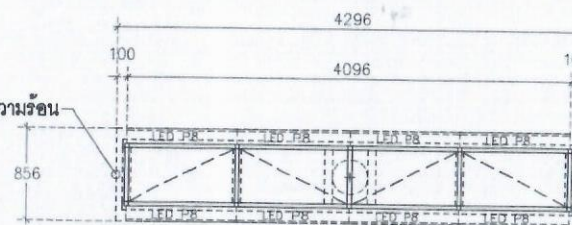
แบบด้านบนกรอบอลูมิเนียมคอมโพสิต SCALE 1 : 50
